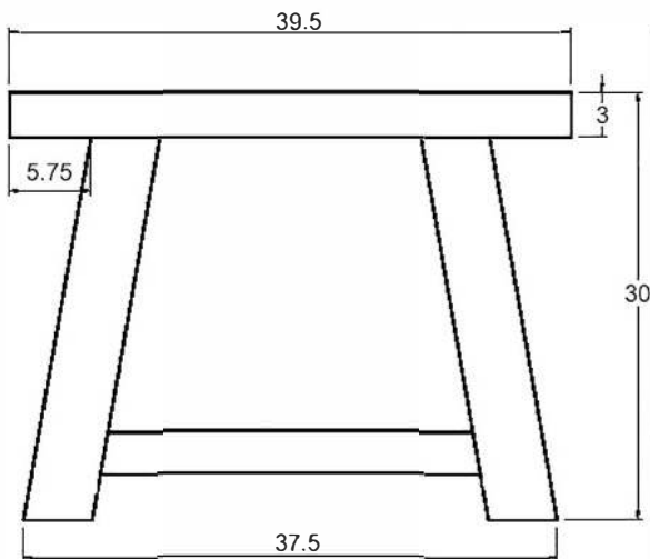
SIDE VIEW/ VUE DE CÔTE/ VISTA LATERAL
